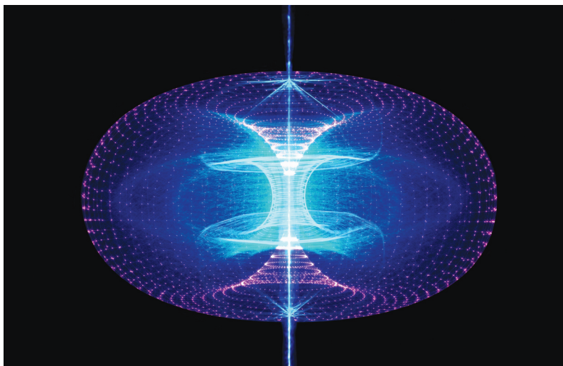
Elektro-magnetisk torusfelt
